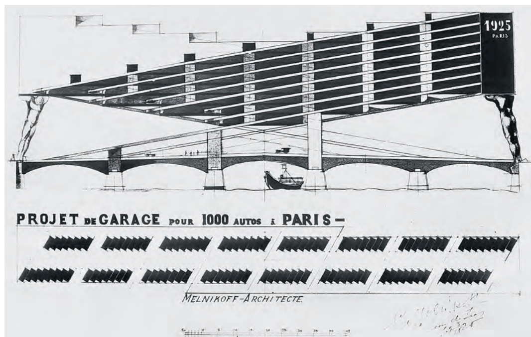
47. Гараж на 1000 машин над мостами Сены в Париже. Фасад. План. 1925 Фоторепродукция В.В.Робинова, 1977 Негатив, ч/б пленка, 13 × 18 ХI-36989
